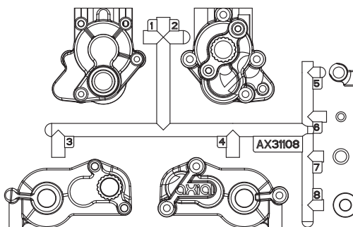
AX31108 (x1) 2-Speed Hi/Low Transmission Case 2-Geschwindigkeiten Hi/Low Getriebeabdeckung Boîtier de la transmission élevé/faible 2 vitesses Scatola trasmissione 2 velocità alta/bassa (HI/LO)
