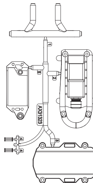
AX31323 (x1) RR10 Electronics Box RR10 Elektronikbox Boîtier des composants électroniques RR10 Scatola elettronica RR10
