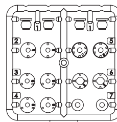
AX80033 (x2) 10mm shock parts tree 10 mm Stoßdämpfer-Teilebaum Arbre des pièces d'amortisseurs 10 mm Set ricambi ammortizzatore 10 mm
